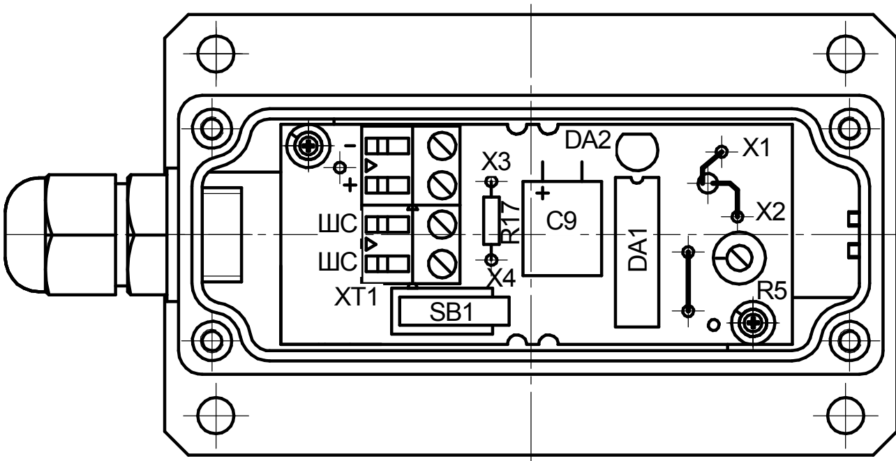
Вид электронного блока без крышки
